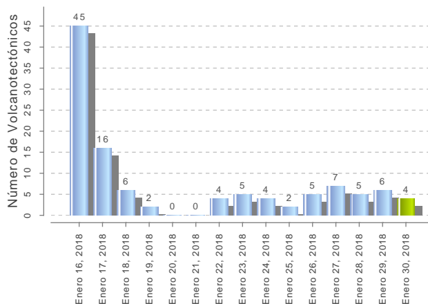
Volcanotectónicos
