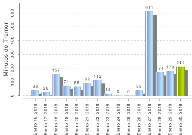
Tremor
