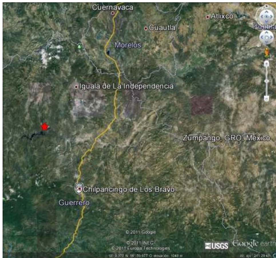
Figura 1. Localización preliminar del sismo del 10 de diciembre de 2011 (Servicio Geológico de los Estados Unidos USGS). La estrella indica la ubicación del epicentro.
