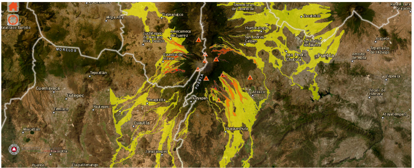
NOTA: Adaptación de los mapas originales publicados por el Instituto de Geofísica de la UNAM.
