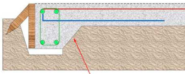
Corte inclinado
