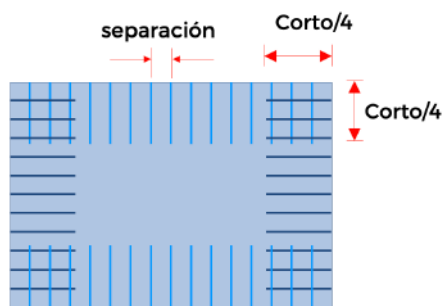
Bastones arriba de bordes
