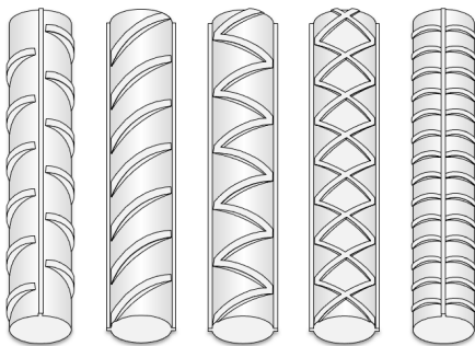
Barras de acero de refuerzo f_y=4200\text{ kg/cm}^2
