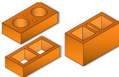
Tabiques huecos
