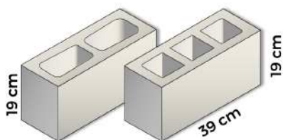
Bloques huecos de concreto
