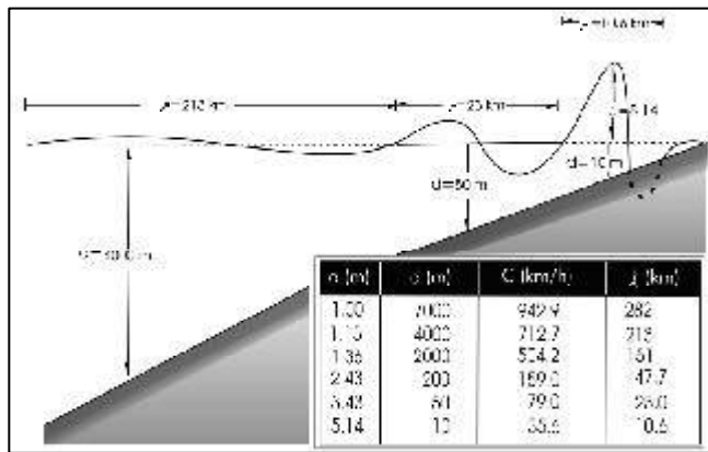
Fig. 13. Disminución de velocidad de fase (c), acortamiento de longitud de onda (b) e incremento de la amplitud (a) de una onda de tsunami de 18 minutos de periodo, por asomeramiento o disminución de la profundidad (d).
